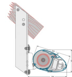
Dachsparrenmontage
