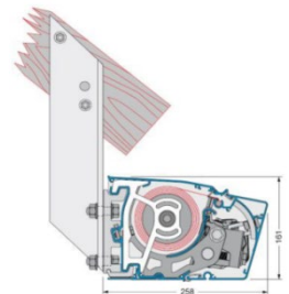
Dachsparrenmontage
