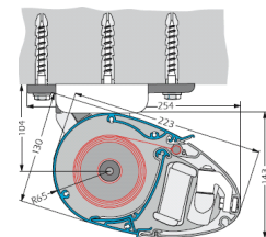
Deckenmontage
