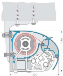
Deckenmontage
