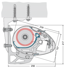
Deckenmontage
