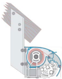
Dachsparrenmontage
