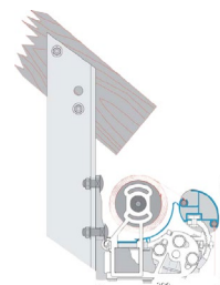
Dachsparrenmontage
